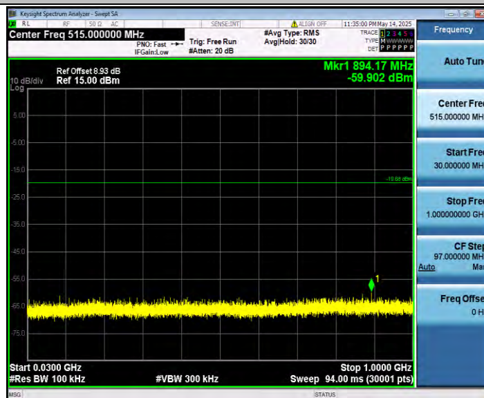
11N20ISO_Ant2_2412_30~1000
