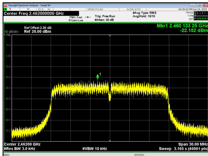
802.11n20 - CH11
