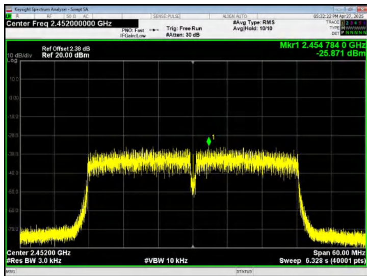
802.11n40 - CH09
