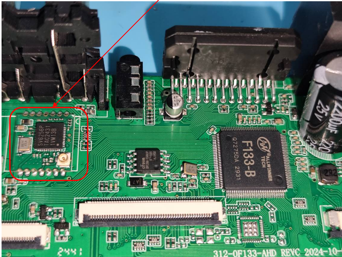
WIFI Module
