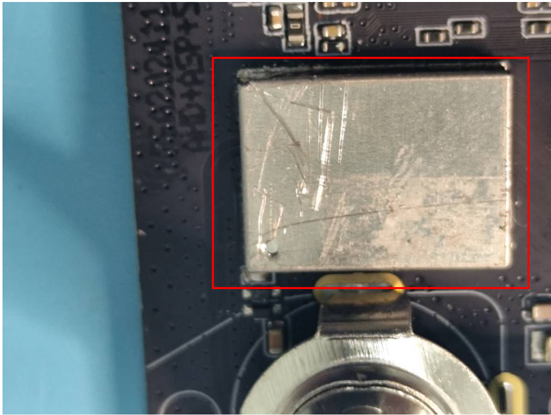
WIFI&BT&GPS&FM Module
