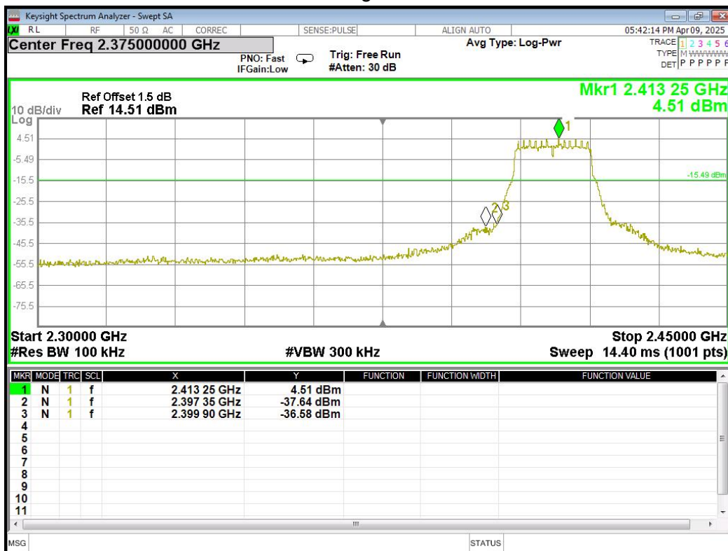
802.11g low CH
