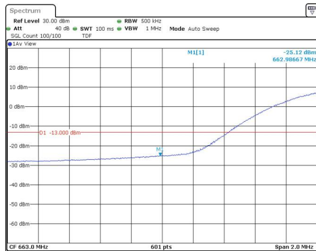
Band71-20MHz-QPSK-133372-1RB#0
