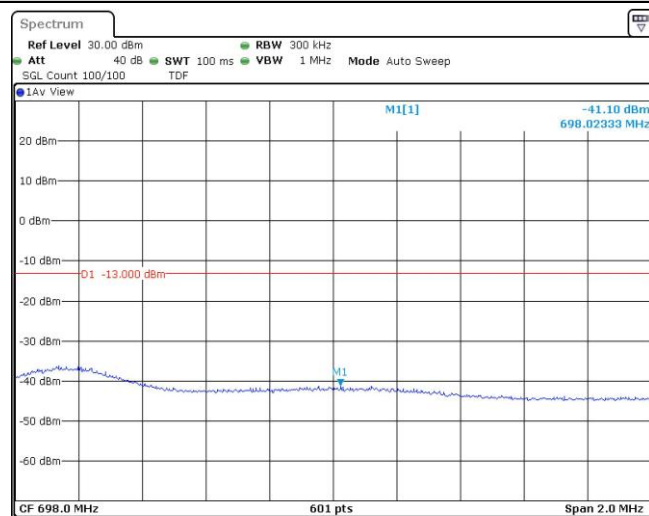
Band71-15MHz-QPSK-133397-1RB#74
