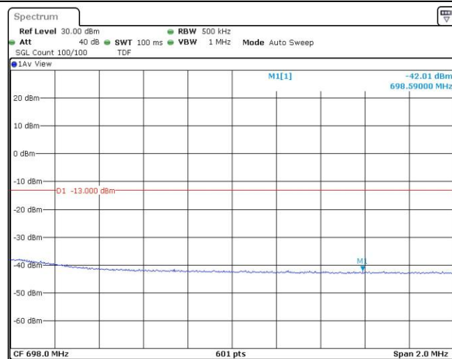
Band71-20MHz-16QAM-133372-1RB#99
