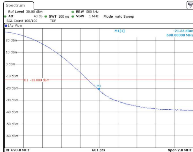
Band71-20MHz-QPSK-133372-100RB#0
