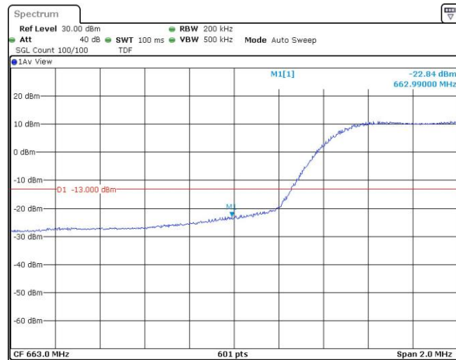
Band71-10MHz-QPSK-133422-1RB#0
