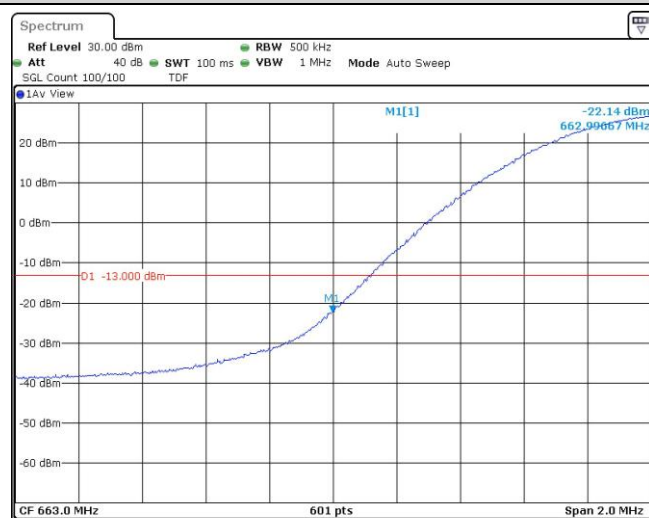
Band71-20MHz-QPSK-133222-1RB#99
