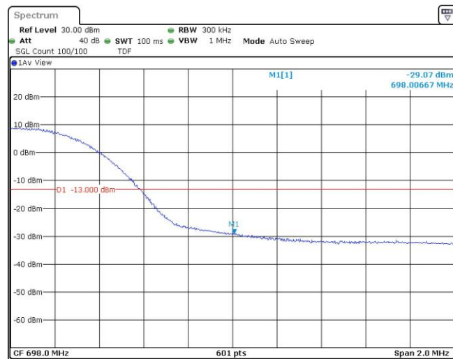
Band71-20MHz-QPSK-133222-1RB#0
