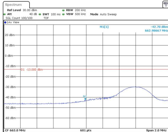
Band71-10MHz-QPSK-133172-50RB#0
