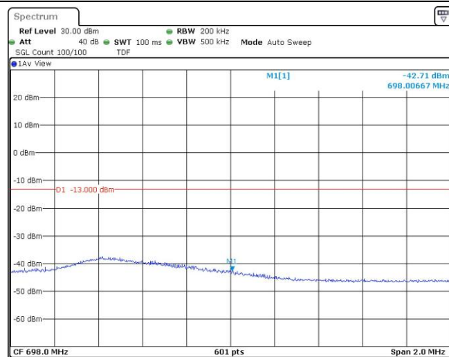
Band71-10MHz-QPSK-133422-1RB#49
