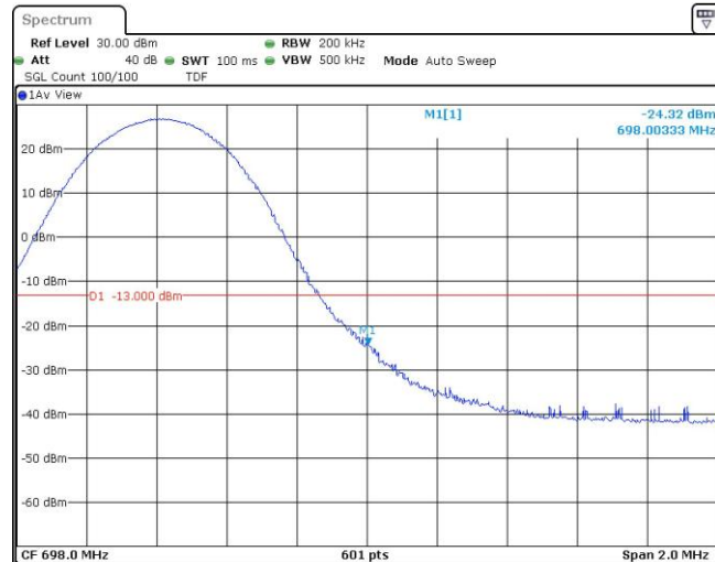
Band71-10MHz-QPSK-133422-50RB#0
