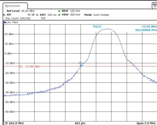
Band71-5MHz-QPSK-133147-1RB#24
