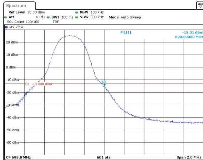
Band71-5MHz-QPSK-133447-25RB#0
