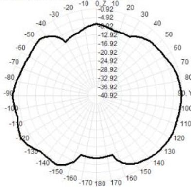
2450.0MHz Total(E2-YZ), Max=-0.92dBi
