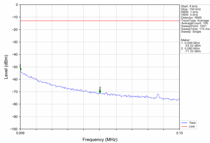
Band2_15MHz_QPSK_LCH_1857.5MHz_RB_1_0_NTNV
