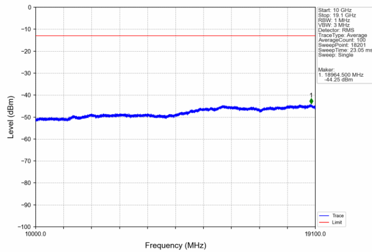
Band2_15MHz_QPSK_MCH_1880MHz_RB_1_0_NTNV
