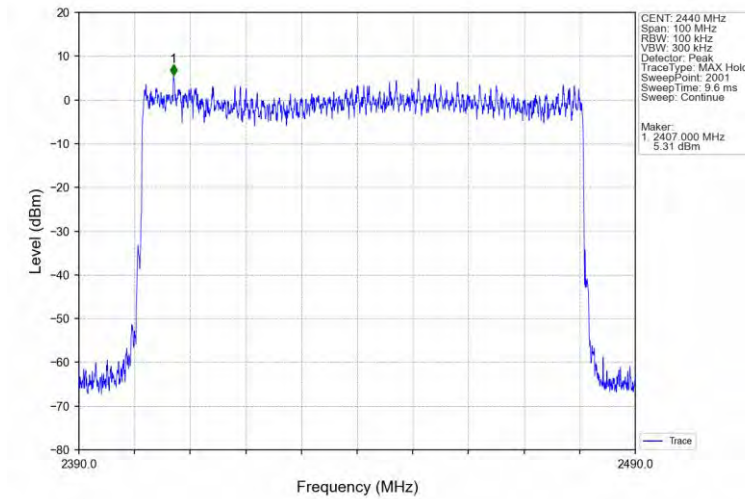
Pi/4DQPSK_2DH5_HOPP_Ant1_NTNV
