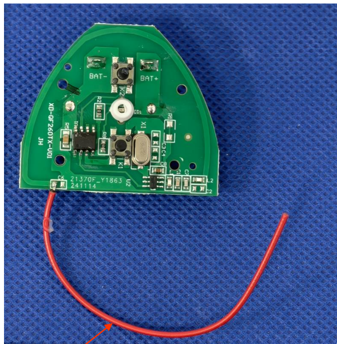
Antenna
