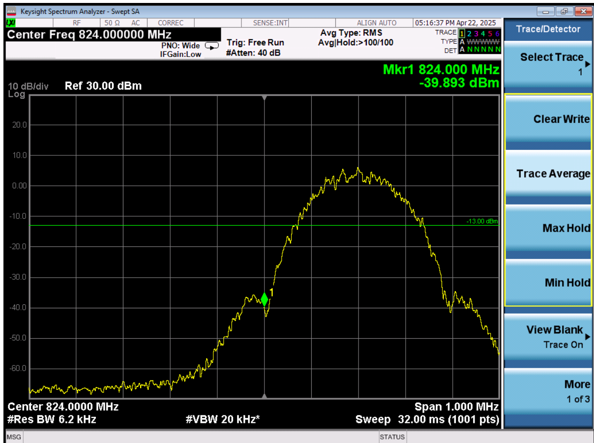
Band edge\GSM850\EGPRS\L
