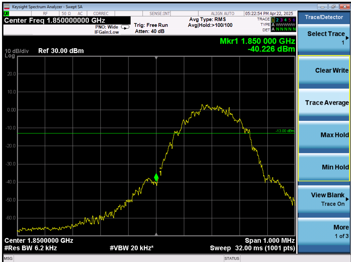
Band edge\GSM1900\EGPRS\L
