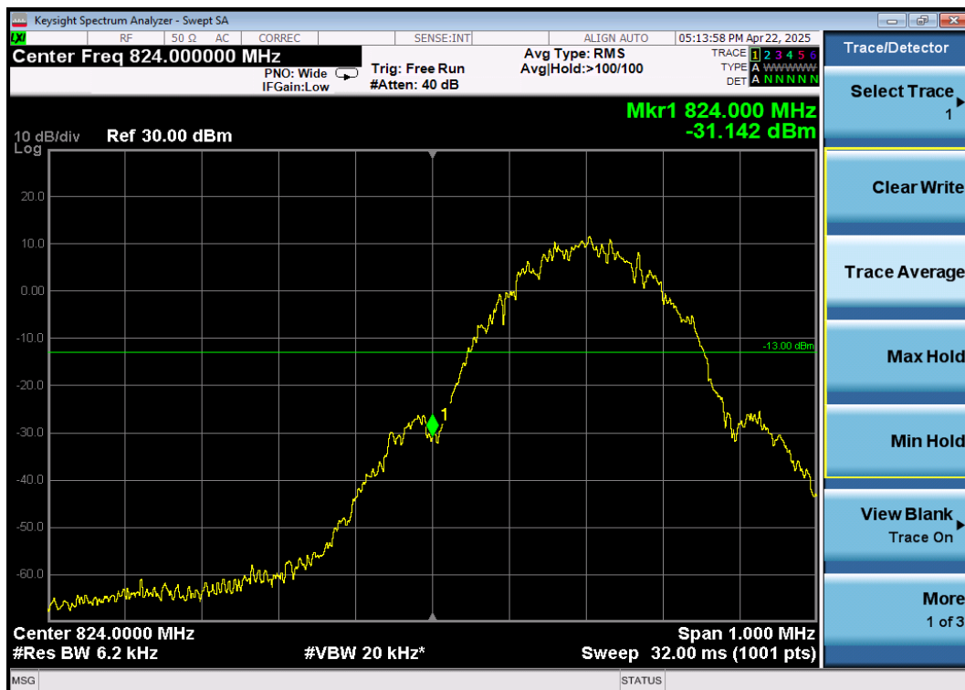
Band edge\GSM850\GPRS\L
