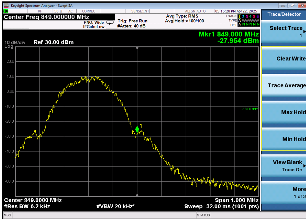
Band edge\GSM850\GPRS\H
