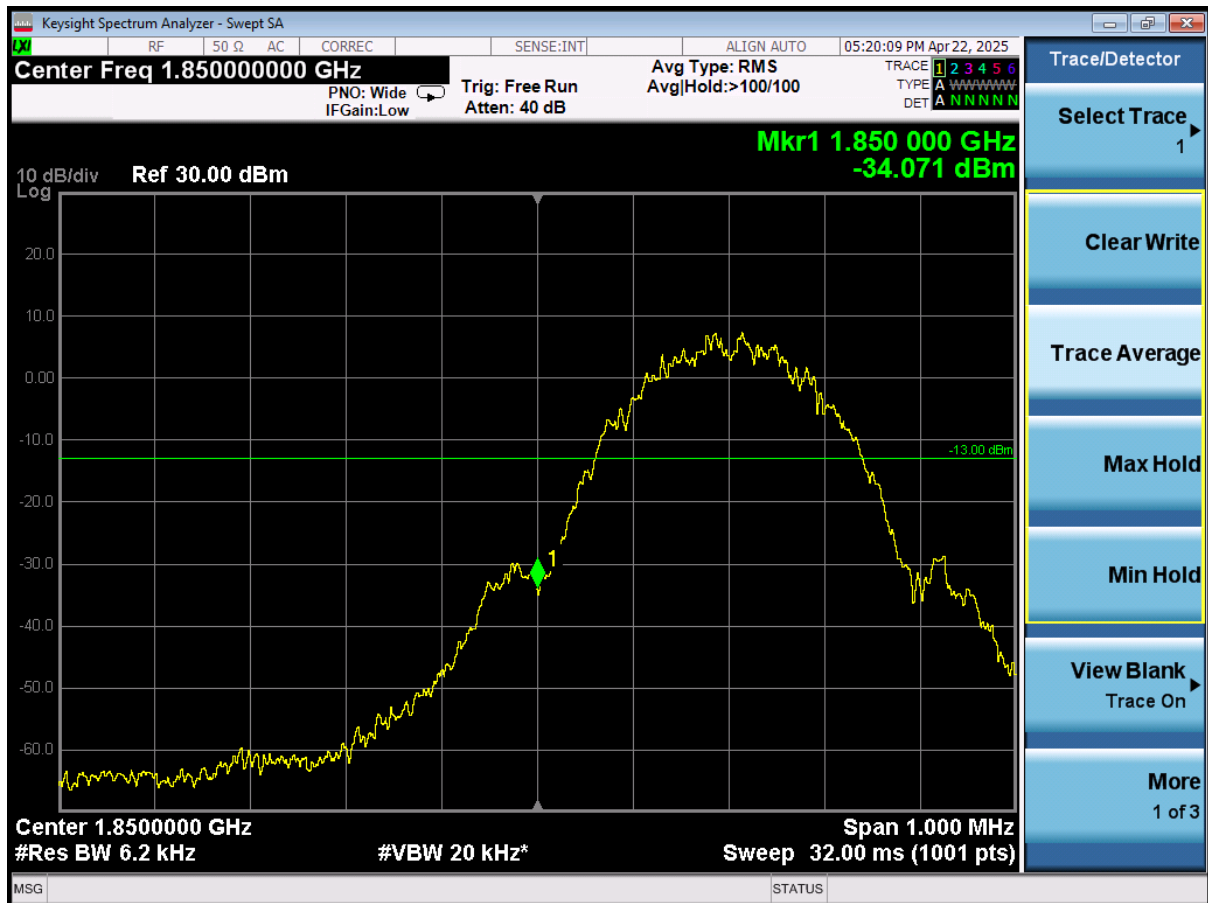
Band edge\GSM1900\GPRS\L
