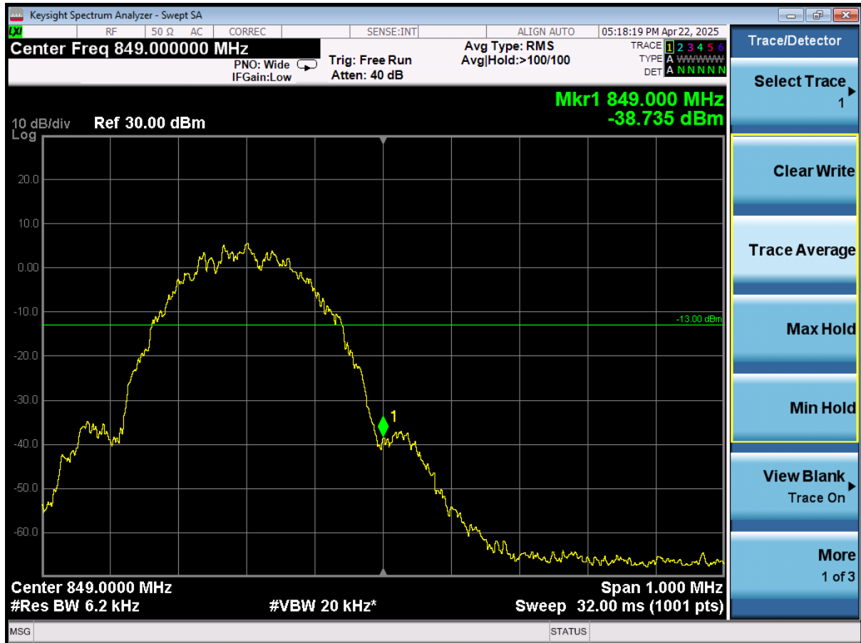
Band edge\GSM850\EGPRS\H
