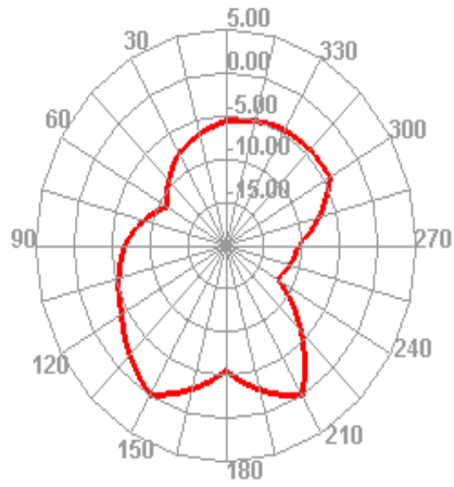
2400.000MHz E1
