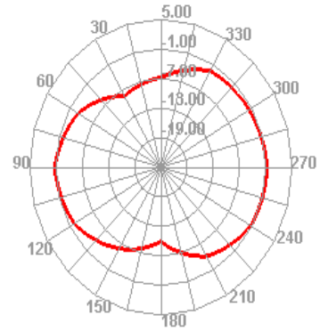
2450.000MHz H
