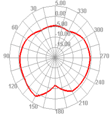
2450.000MHz E2
