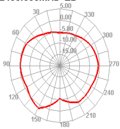
2400.000MHz E2
