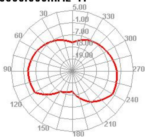
5500.000MHz H
