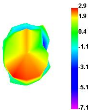
5500.000MHz E1
