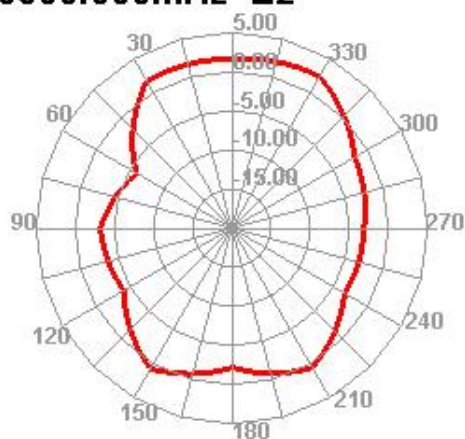
5500.000MHz E2
