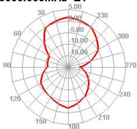
5500.000MHz E1
