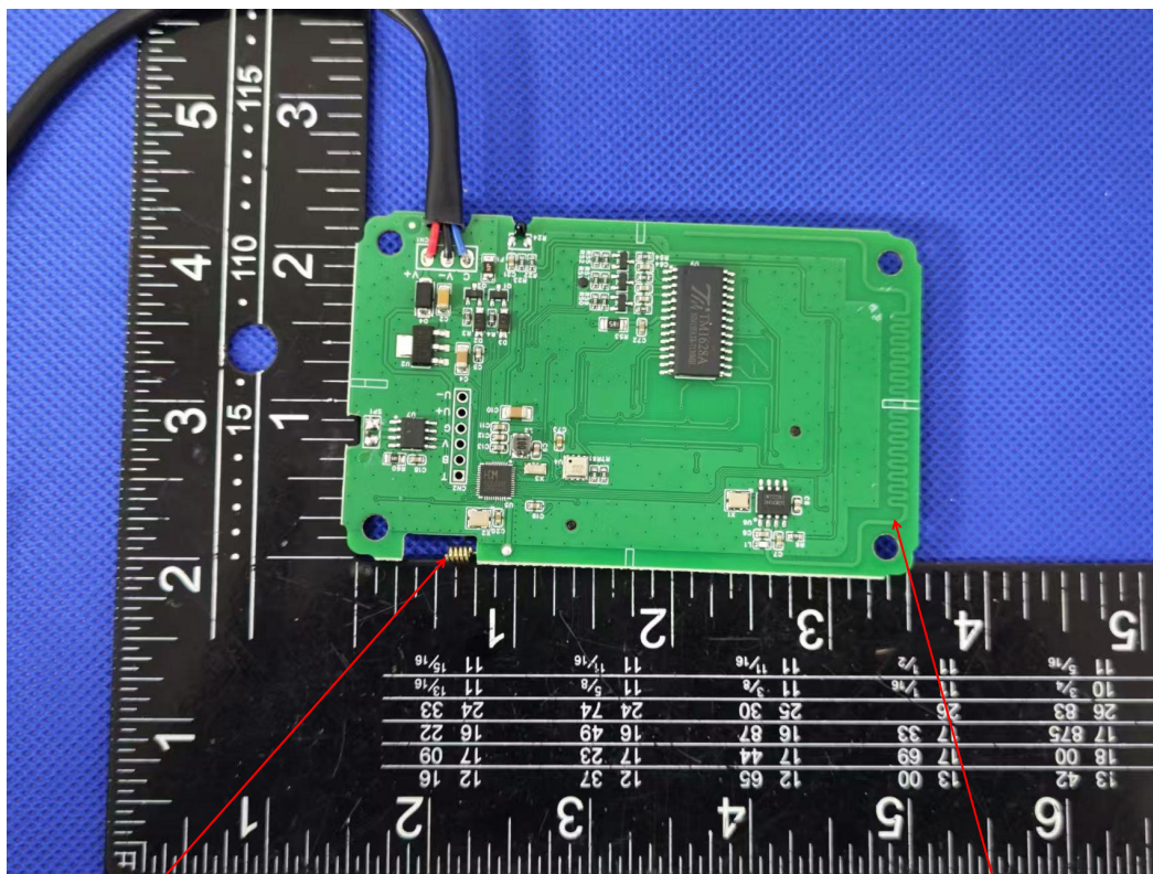
BLE Spring antenna
