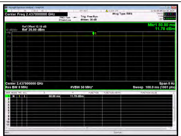
802.11b 2437MHz
