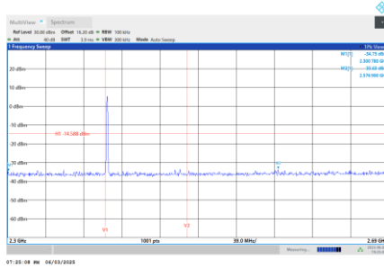
Bandedge-CH00
