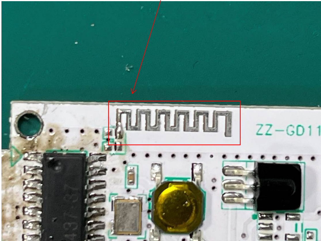
BLE Ant
