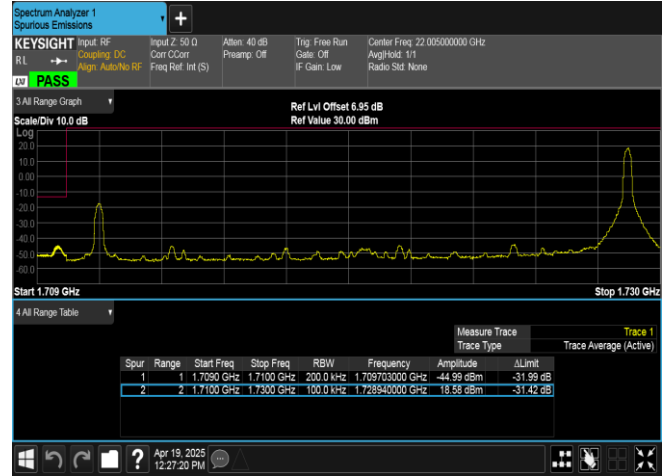
Band66-20MHz-QPSK-132072-1RB#99-PASS
