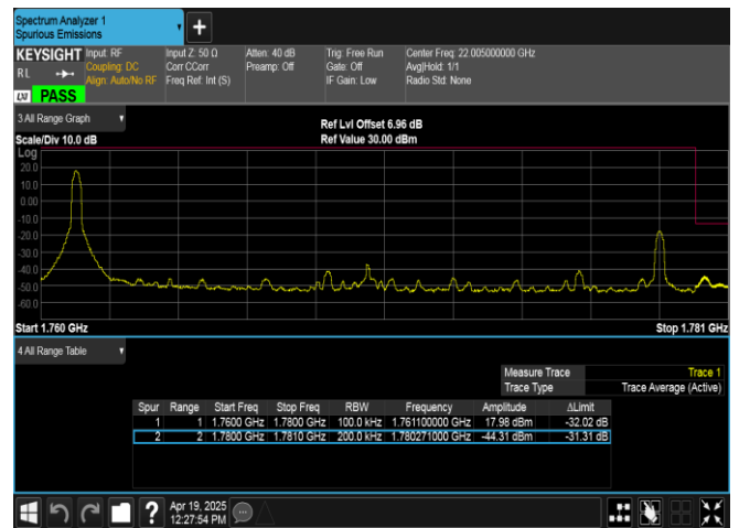
Band66-20MHz-QPSK-132572-1RB#0-PASS
