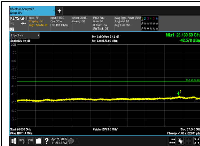
Band41-20MHz-QPSK-41490-100RB#0-20000~27000-PASS
