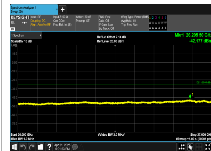
Band41-15MHz-16QAM-41515-1RB#74-20000~27000-PASS
