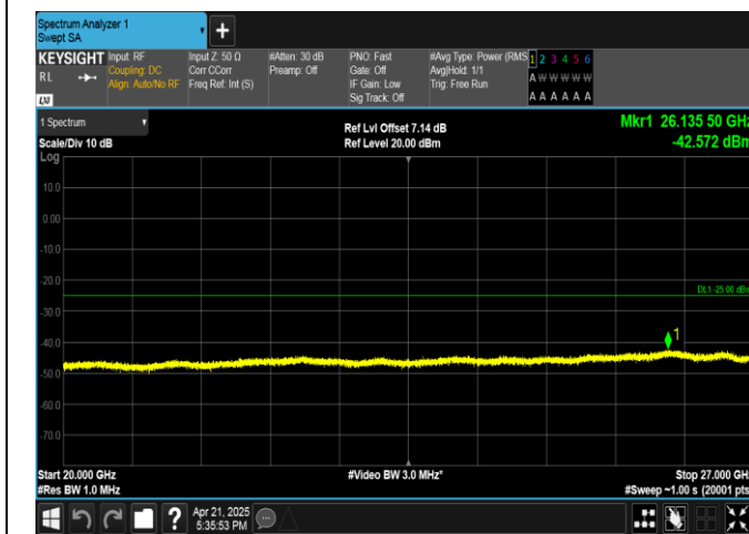
Band41-20MHz-QPSK-41490-1RB#0-20000~27000-PASS
