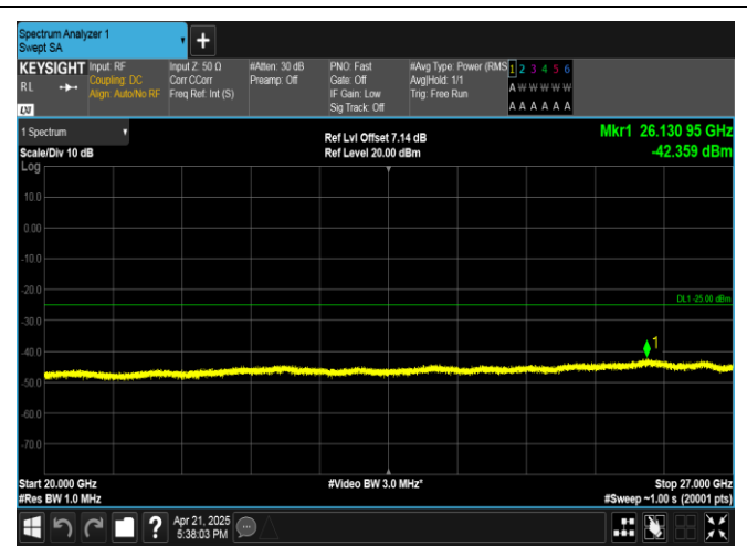
Band41-20MHz-QPSK-41490-1RB#99-20000~27000-PASS
