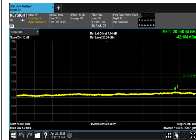
Band41-20MHz-QPSK-39750-1RB#0-20000~27000-PASS
