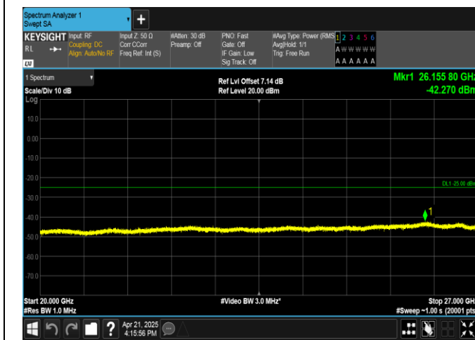
Band41-10MHz-QPSK-41540-1RB#0-20000~27000-PASS
