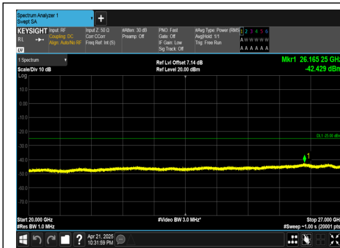
Band41-10MHz-QPSK-41540-50RB#0-20000~27000-PASS
