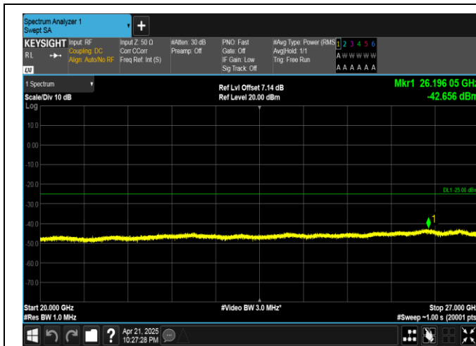
Band41-10MHz-QPSK-39700-50RB#0-20000~27000-PASS
