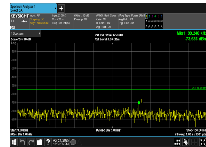
Band41-10MHz-QPSK-41540-50RB#0-0.009~0.15-PASS
