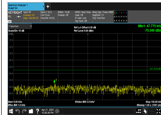
Band41-10MHz-QPSK-39700-50RB#0-0.009~0.15-PASS
