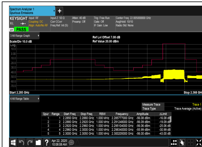
Band40(2350-2360)-10MHz-QPSK-39200-50RB#0-PASS
