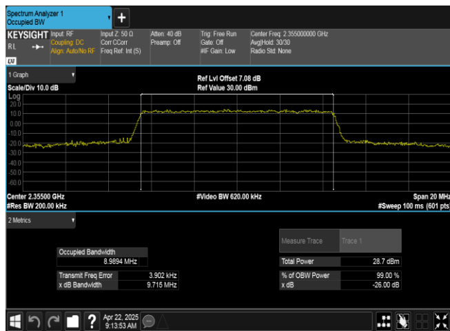
Band40(2350-2360)-10MHz-QPSK-39200-50RB#0-PASS
