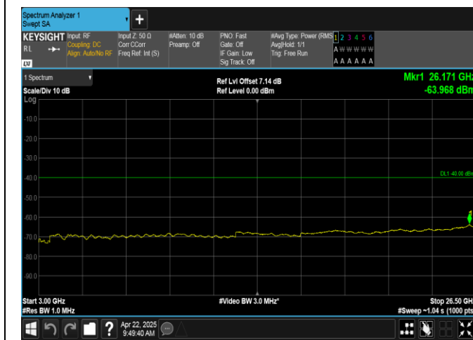
Band40(2305-2315)-10MHz-QPSK-38750-50RB#0-3000~26500-PASS
