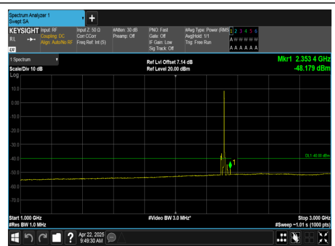
Band40(2305-2315)-10MHz-QPSK-38750-50RB#0-1000~3000-PASS
