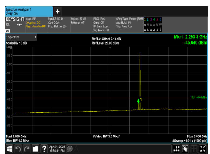
Band40(2305-2315)-5MHz-QPSK-38725-25RB#0-1000~3000-PASS
