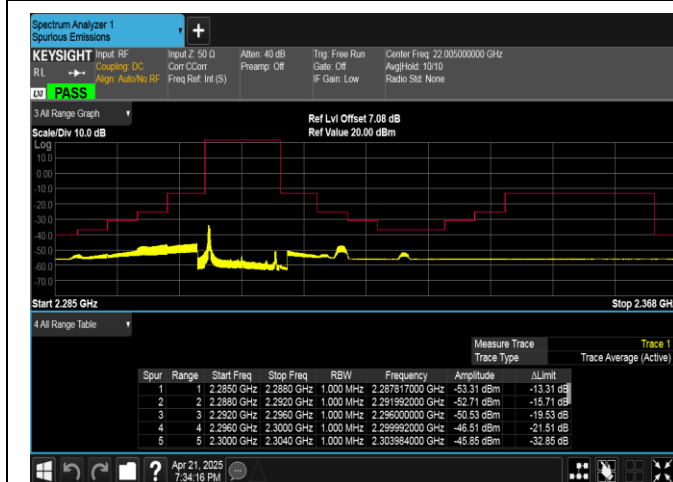
Band40(2305-2315)-10MHz-QPSK-38750-1RB#0-PASS
