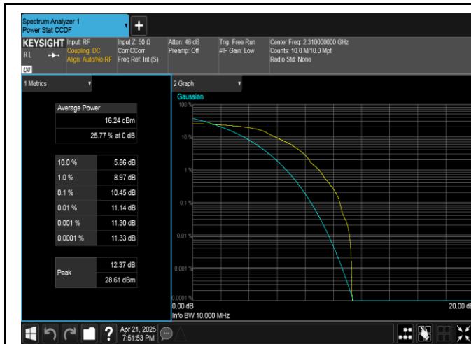
Band40(2305-2315)-10MHz-QPSK-38750-1RB#0-PASS
