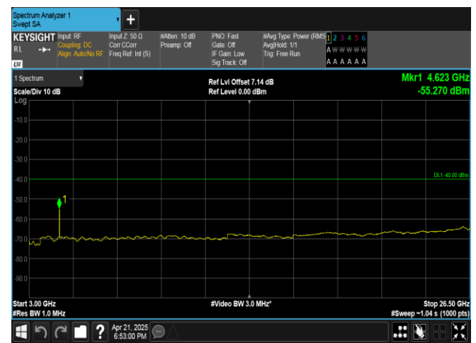
Band40(2305-2315)-5MHz-QPSK-38725-1RB#24-3000~26500-PASS
