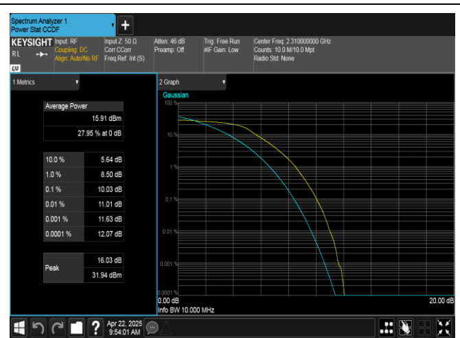
Band40(2305-2315)-10MHz-QPSK-38750-50RB#0-PASS
