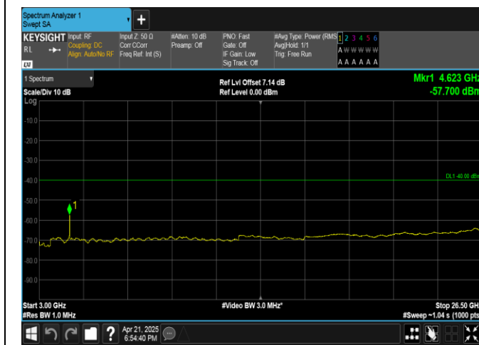
Band40(2305-2315)-5MHz-QPSK-38725-25RB#0-3000~26500-PASS
