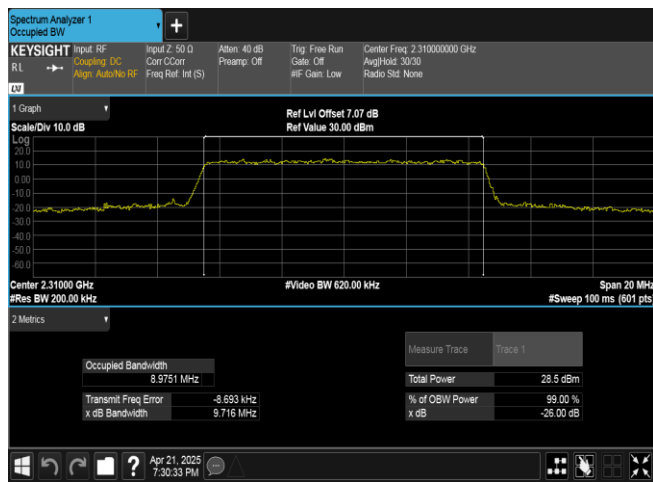
Band40(2305-2315)-10MHz-QPSK-38750-50RB#0-PASS
