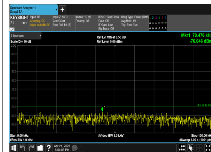
Band40(2305-2315)-5MHz-QPSK-38725-25RB#0-0.009~0.15-PASS
