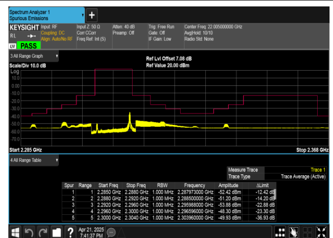
Band40(2305-2315)-10MHz-QPSK-38750-1RB#49-PASS
