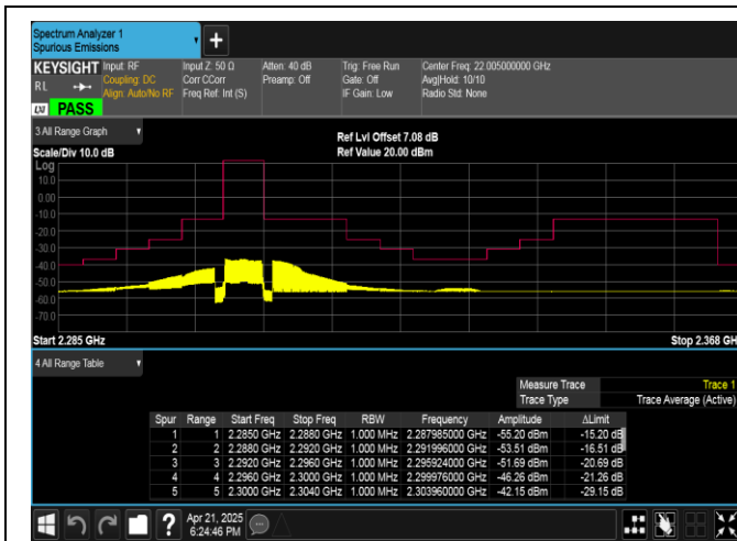
Band40(2305-2315)-5MHz-QPSK-38725-25RB#0-PASS
