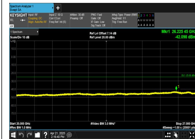
Band38-20MHz-QPSK-37850-1RB#0-20000~27000-PASS
