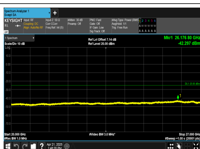
Band38-15MHz-OPSK-38175-1RB#74-20000~27000-PASS
