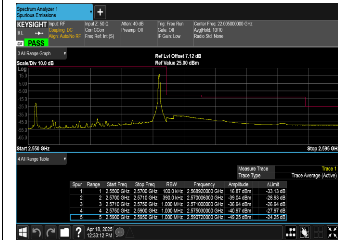
Band7-20MHz-QPSK-21350-1RB#99-PASS
