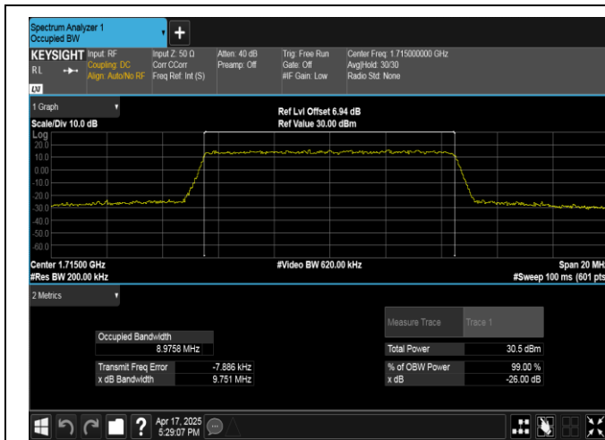
Band4-10MHz-QPSK-20000-50RB#0-PASS
