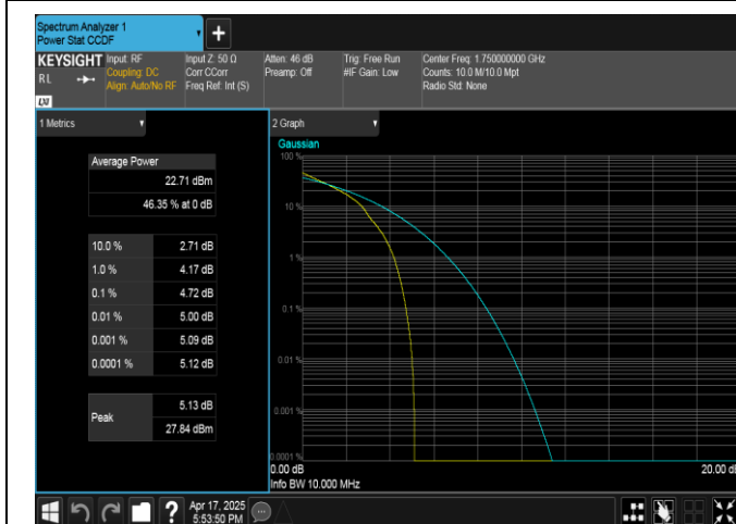
Band4-10MHz-QPSK-20350-1RB#0-PASS
