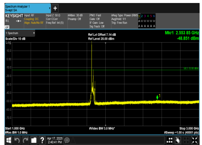
Band2-20MHz-QPSK-18700-1RB#0-1000~3000-PASS
