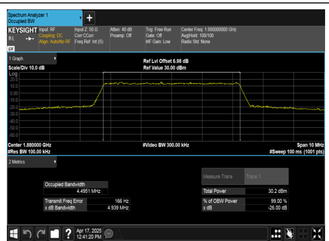
Band2-5MHz-QPSK-18900-25RB#0-PASS
