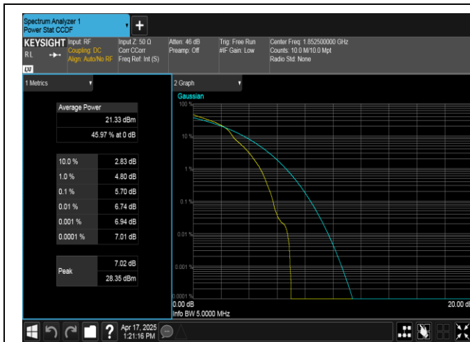
Band2-5MHz-16QAM-18625-1RB#0-PASS
