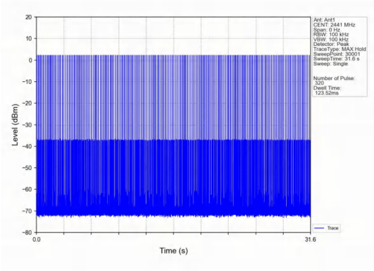
Pi/4DQPSK_2DH1_HOPP_Ant1_NTNV
