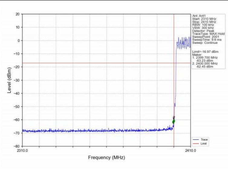
Pi/4DQPSK_2DH5_HOPP_Ant1_NTNV
