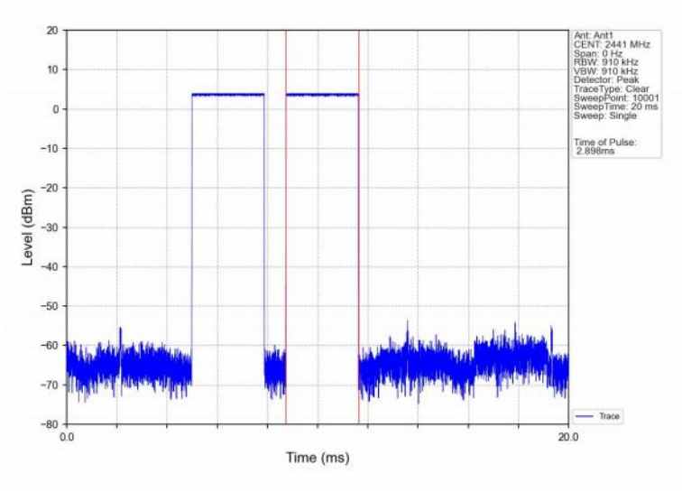
GFSK_DH5_HOPP_Ant1_NTNV
