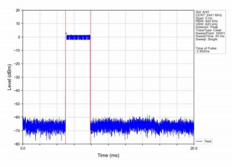
Pi/4DQPSK_2DH5_HOPP_Ant1_NTNV
