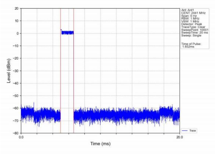
Pi/4DQPSK_2DH3_HOPP_Ant1_NTNV
