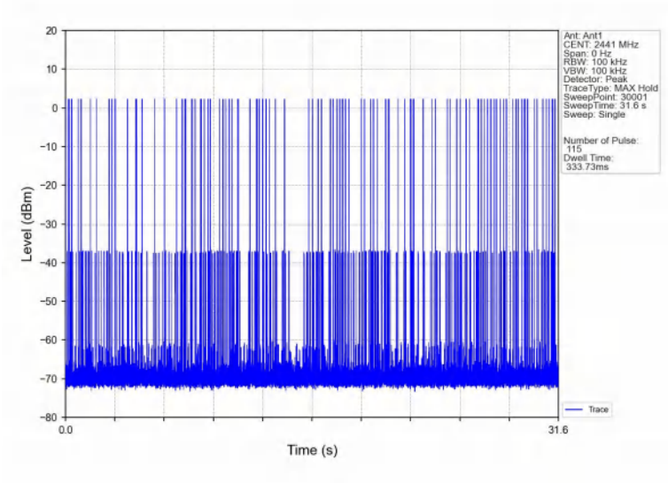
Pi/4DQPSK_2DH5_HOPP_Ant1_NTNV
