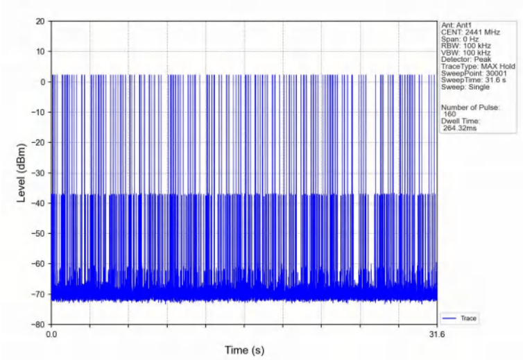
Pi/4DQPSK_2DH3_HOPP_Ant1_NTNV
