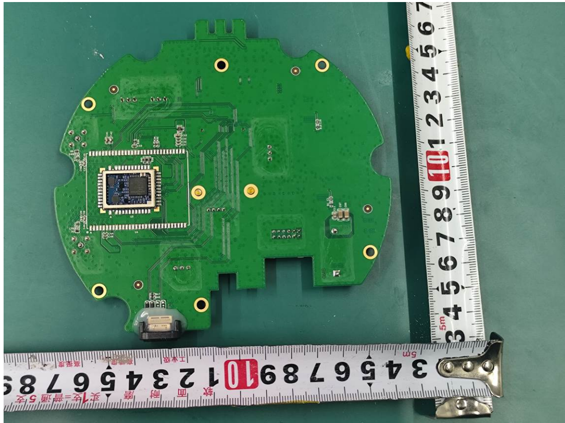
GNSS Module
