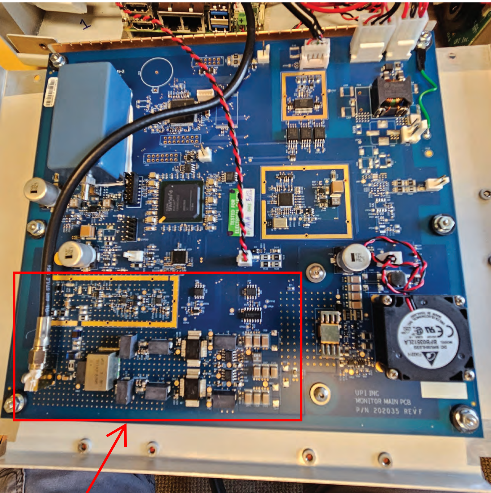
RFID Radio
