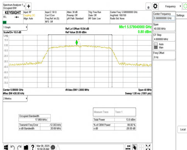
11N20MIMO_Ant1_5580
