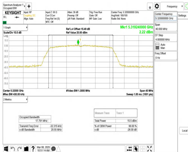
11N20MIMO_Ant1_5320
