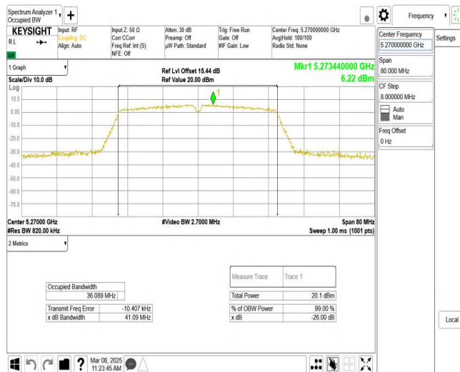
11N40MIMO_Ant1_5270
