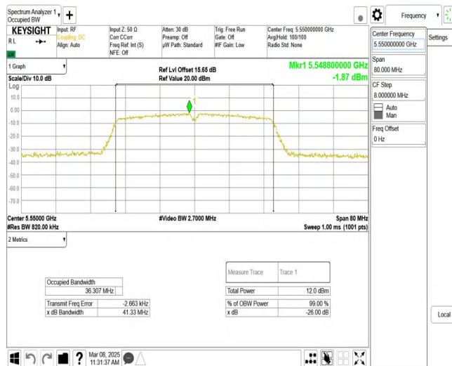
11N40MIMO_Ant1_5550
