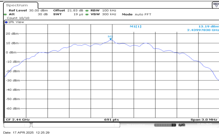
BLE 2M Ant1 2440 0-Reference
