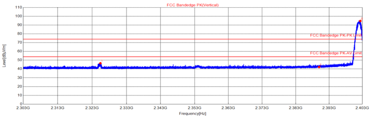
BLE_1M_2402_Ant1/ Vertical
