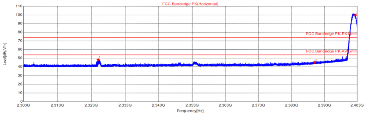
BLE_1M_2402_Ant1/ Horizontal
