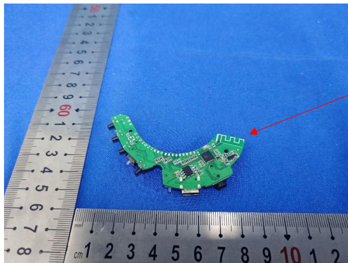
Antenna
