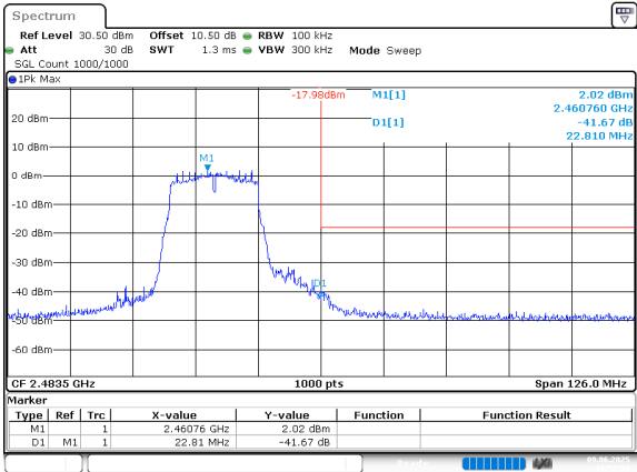
802.11n20_2462MHz_Chain 1
