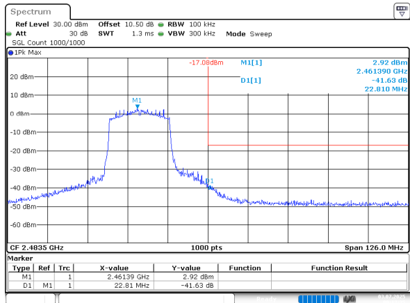
802.11ax20_2462MHz_Chain 1
