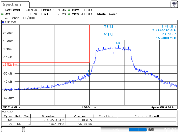
802.11n20_2412MHz_Chain 1
