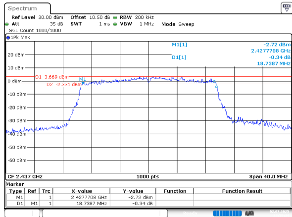
802.11ax20_2437MHz_Chain 0
