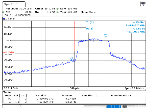
802.11ax20_2412MHz_Chain 1
