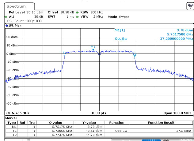
802.11n40_5755MHz_Chain 0
