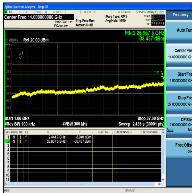
SRD-Ant1-2445-1000~27000-PASS
