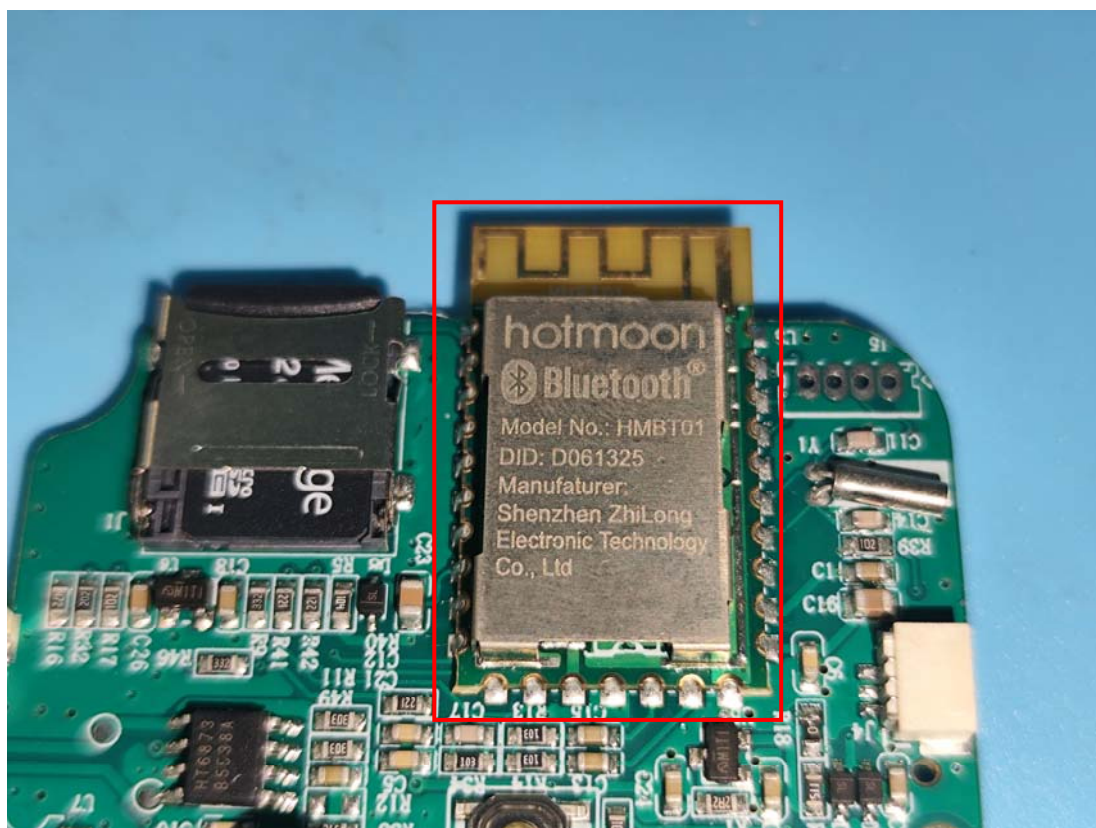
RF Module
