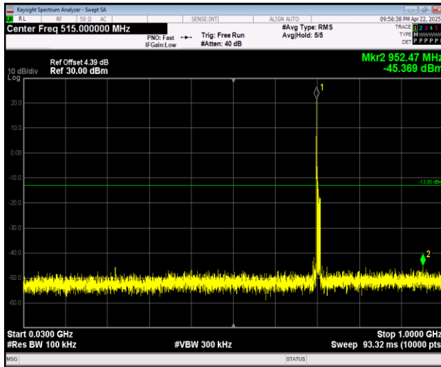
Band25-1.4MHz-QPSK-26047-1RB#0-Range1:30~10 00MHz
