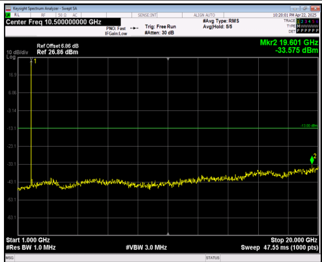
Band25-1.4MHz-QPSK-26365-1RB#0-Range2:1000~ 20000MHz
