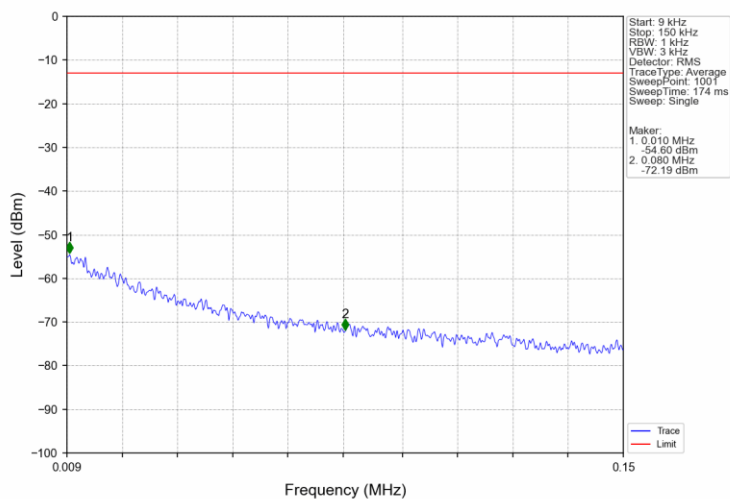
Band25_20MHz_QPSK_LCH_1860MHz_RB_1_0_NTNV
