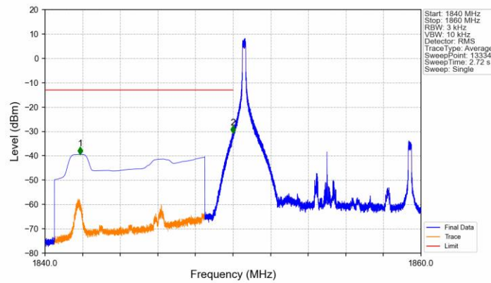
Band25_10MHz_QPSK_LCH_1855MHz_RB_1_0_NTNV
