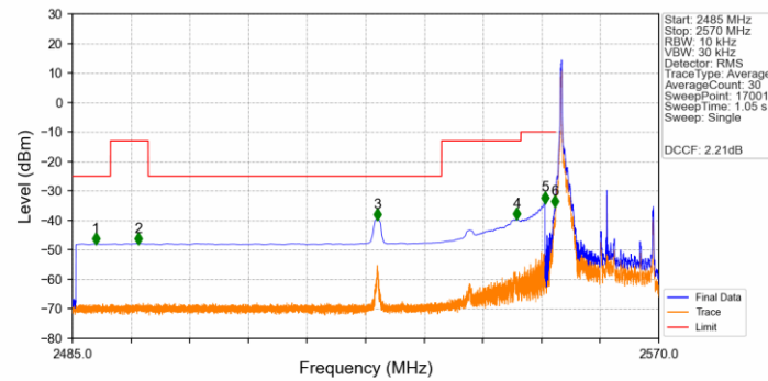
Band41_15MHz_QPSK_LCH_2562.5MHz_RB_1_0_NTNV
