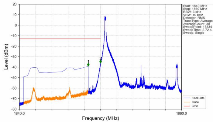
Band2_10MHz_QPSK_LCH_1855MHz_RB 1 0 NTN
