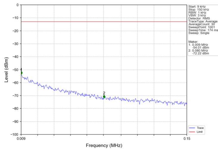
Band2_10MHz_QPSK_LCH_1855MHz_RB 1 0 NTN
